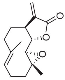
小白菊内酯(Parthenolide)
